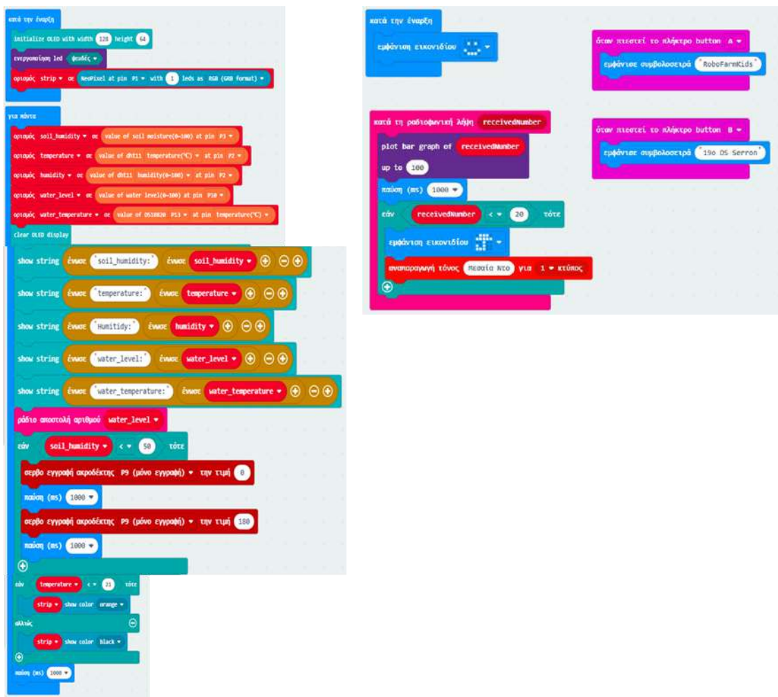
Εικόνα 17. Κώδικας 2ου microbit
